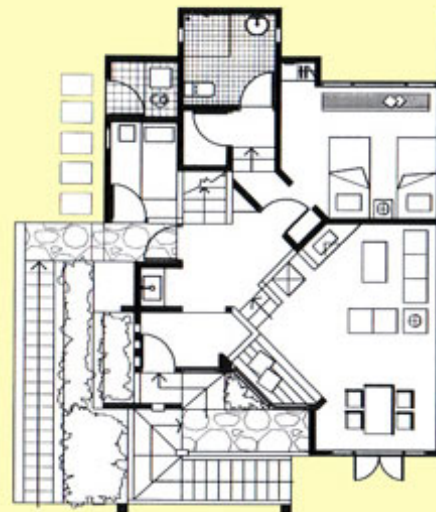
LANTAI BAWAH
